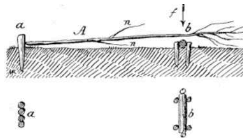
Fig. 22. — Coupe en élévation et plan d'un billot pour la préparation des bois.
